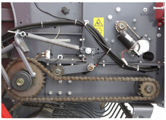
ПРИВОД С ОБЕИХ СТОРОН МАШИНЫ
